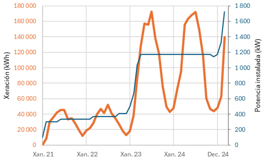
Ilustración 21. Enerxía producida e potencia fotovoltaica instalada
