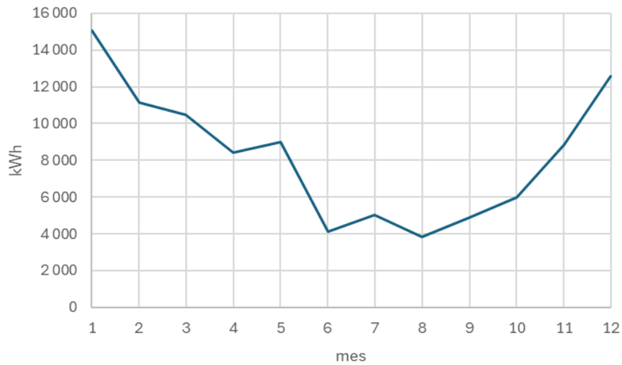
Ilustración 34. Consumo de enerxía eléctrica da xeotermia da biblioteca central (campus de Vigo)
