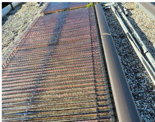
Ilustración 35. Instalación solar térmica con tubos de baleiro na Ecimat
