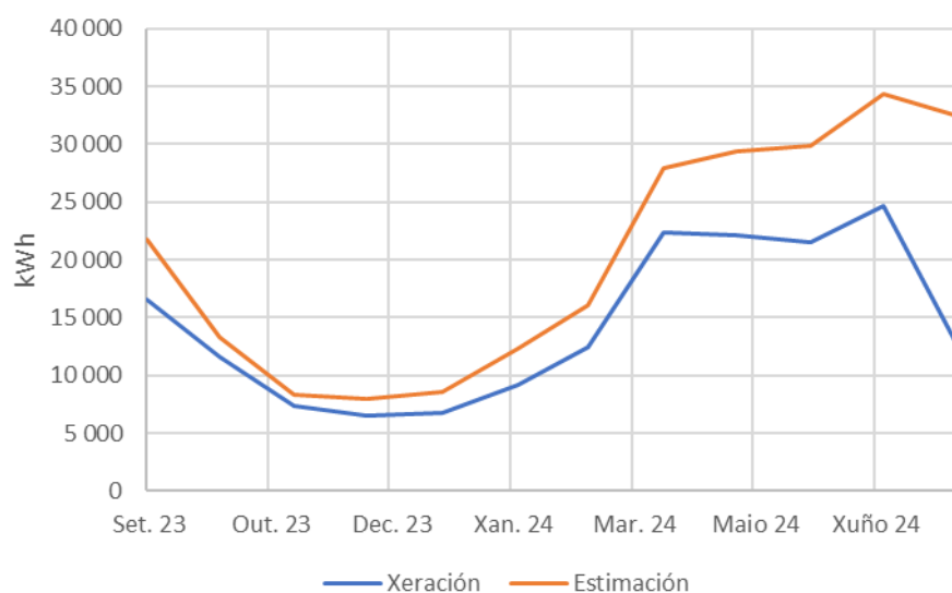
Ilustración 25. Enerxía xerada e estimación da enerxía que se podería xerar na instalación da Escola de Enxeñaría Industrial, sede campus (200 kW)
