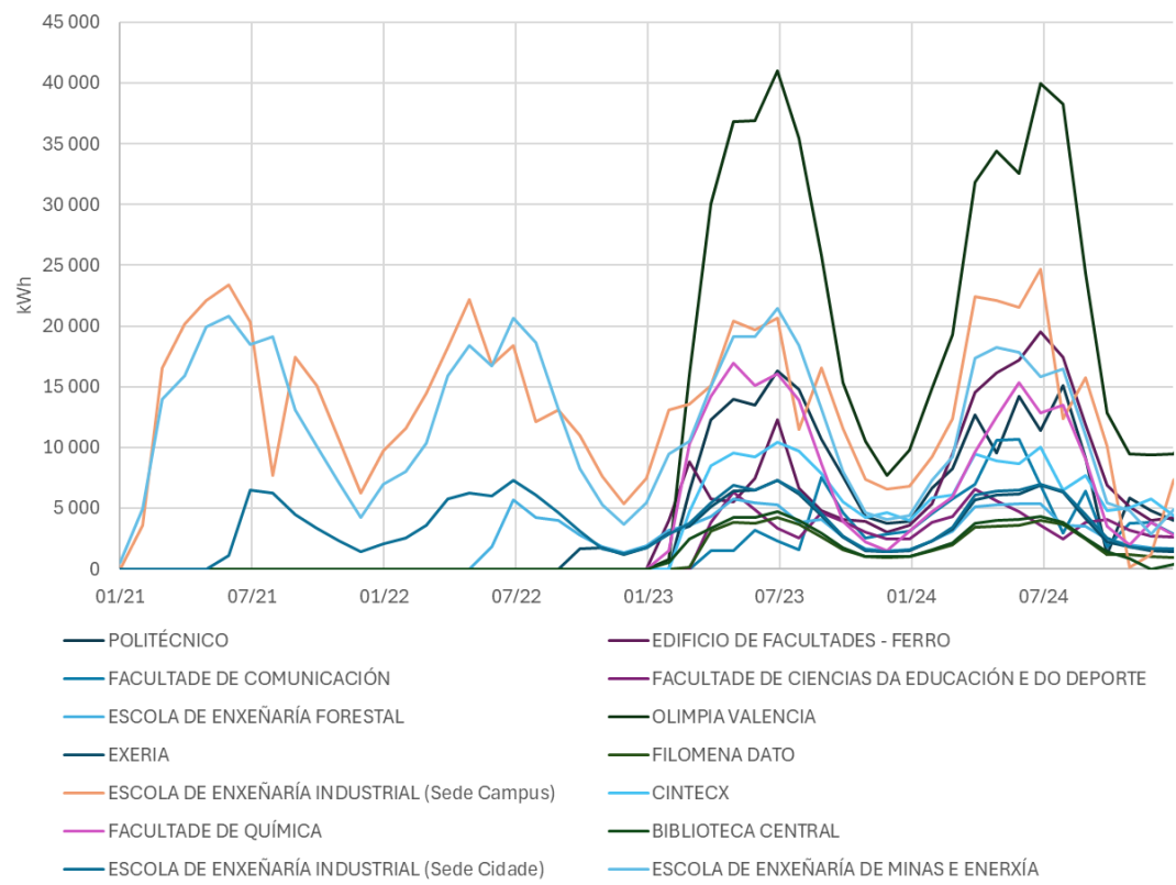
Ilustración 22. Producción fotovoltaica mensual
